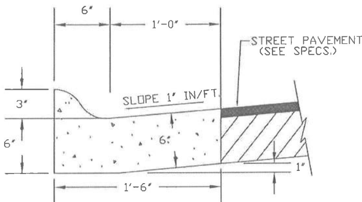
ROLL CURB & GUTTER
