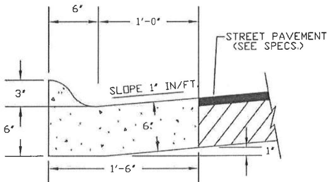
ROLL CURB & GUTTER
